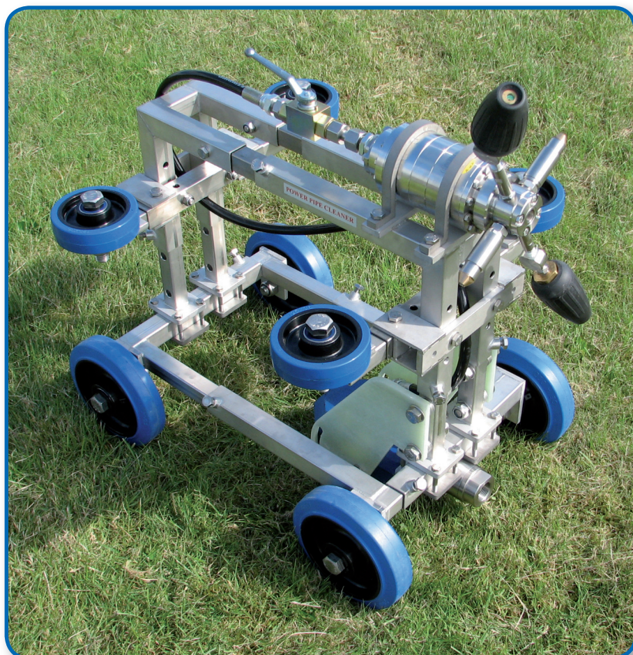
Til rensning af regnvandskanaler og rør fra DN800 til DN3000.
